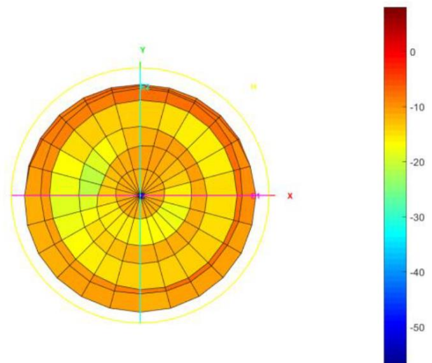
Total_3D_Front View_1.57542GHz
