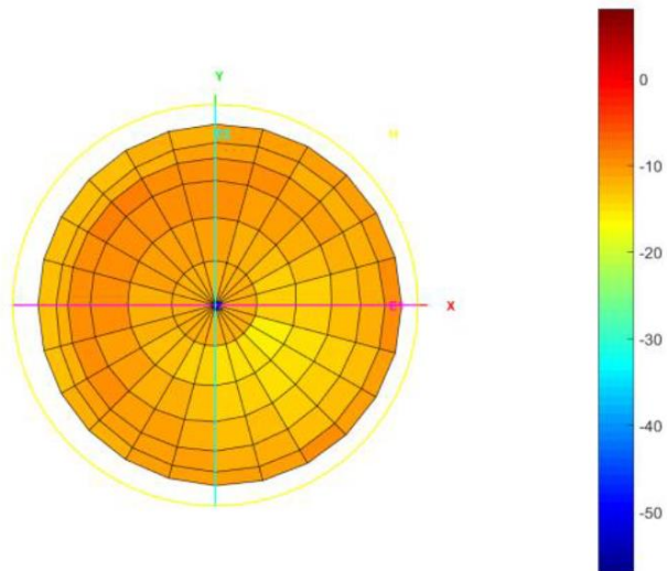
Total_3D_Front View_698MHz
