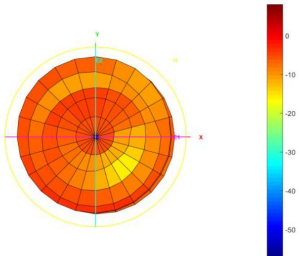
Total_3D_Front View_960MHz
